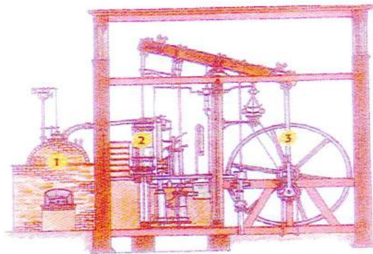
De stoommachine van James Watt
