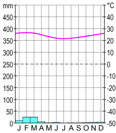
klimaatdiagram van Piura
