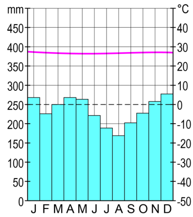
klimaatdiagram van Iquitos
